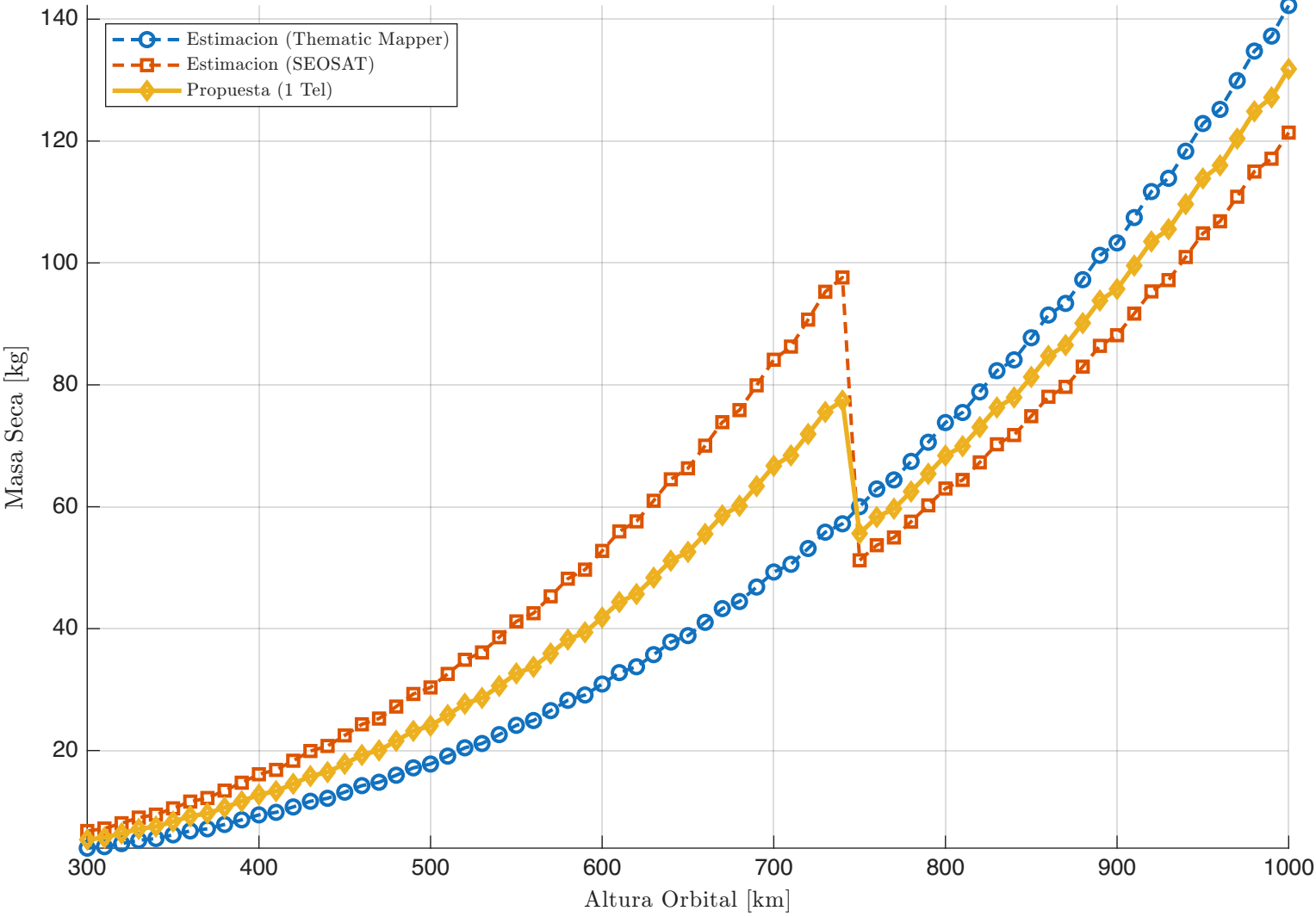
Comparativa de Masa Seca vs. Altura Config: 1 Sat, 1 Tel, Det 1, Cassegrain
